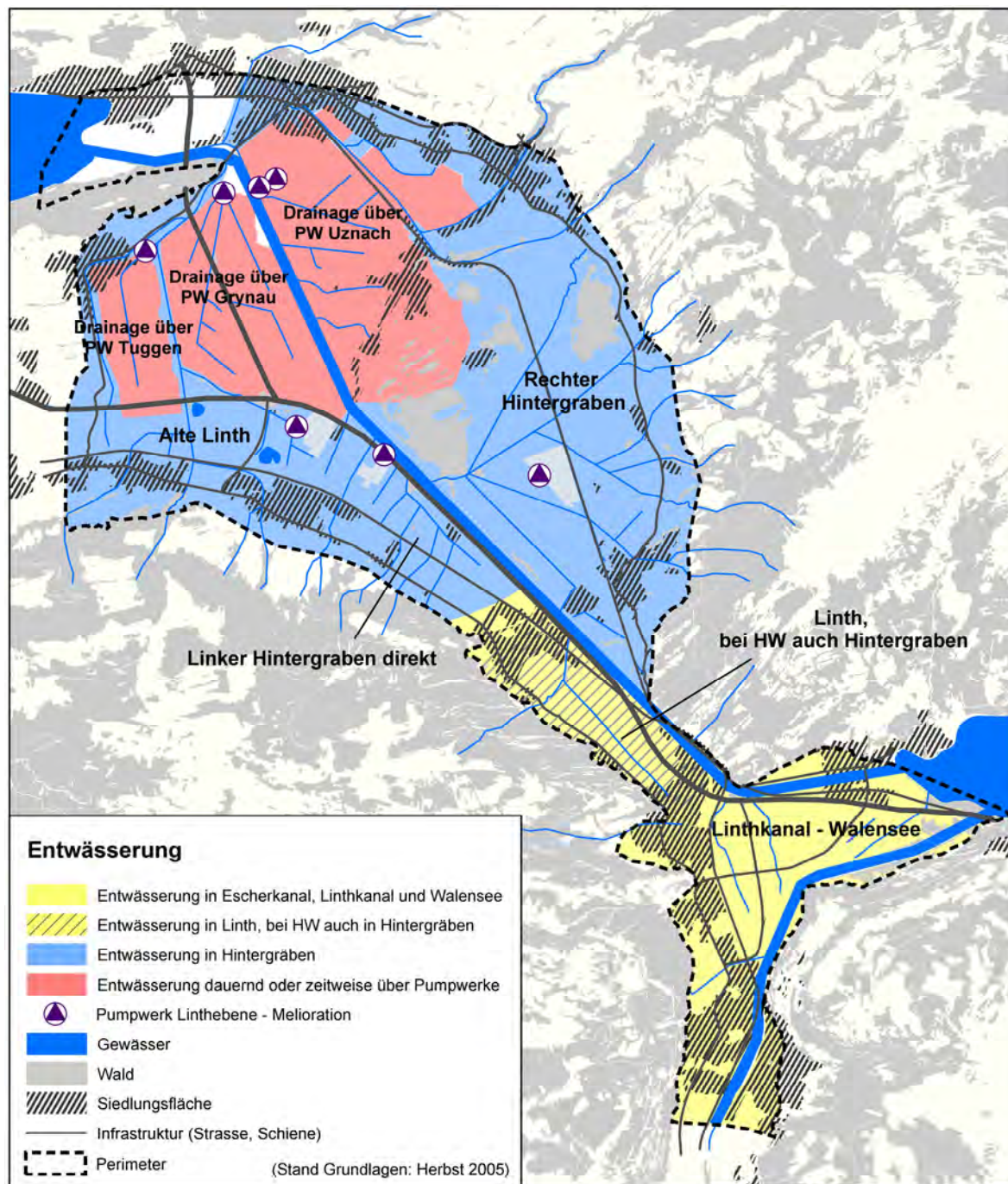
Abb. 3-1: Generalisierte Darstellung der hydrologischen Ebenen im Linthgebiet unter dem Gesichtspunkt der Entwässerung. Weitere kleine Gebiete, in denen die Abführung des Wassers nur über Pumpen möglich ist, befinden sich in den Gemeinden Reichenburg und Schänis (→ TP 2).
